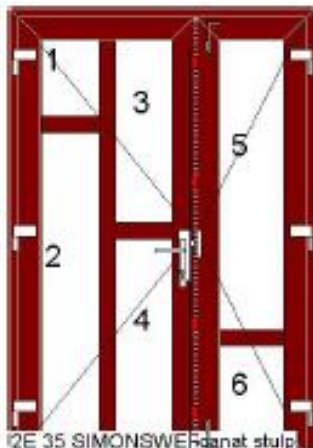
JE35 SIMONSWERK
